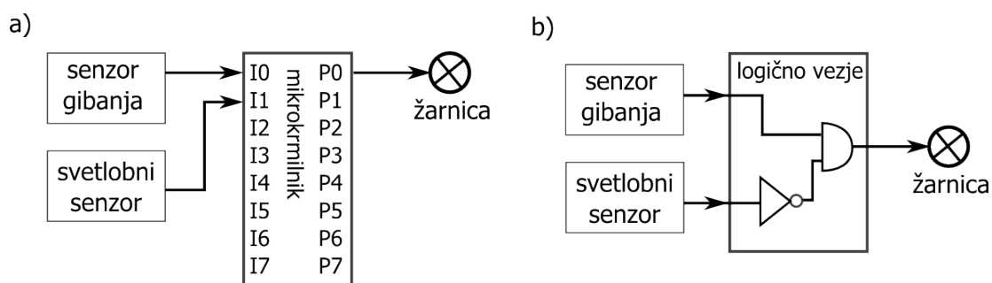
Slika 1.7: Senzor gibanja v temi: a) z mikrokrmilnikom in b) z logičnim vezjem
