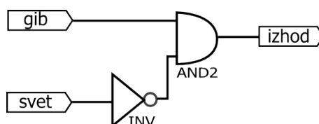
Slika 1.8: Shema logičnega vezja za senzor gibanja
